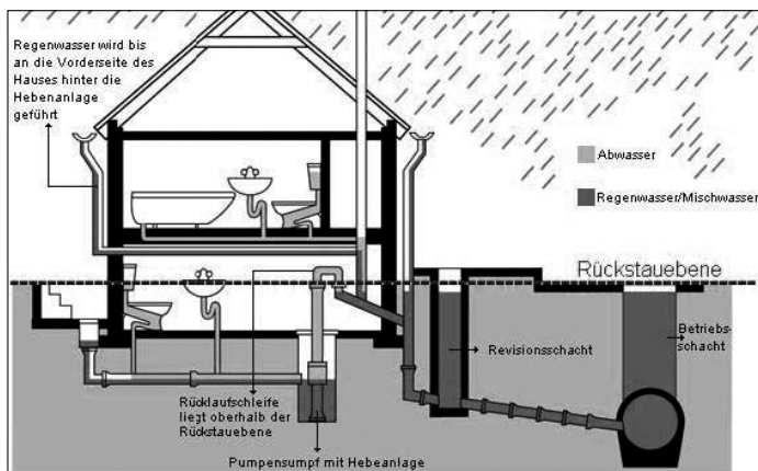
4.1 Hebeanlagen
