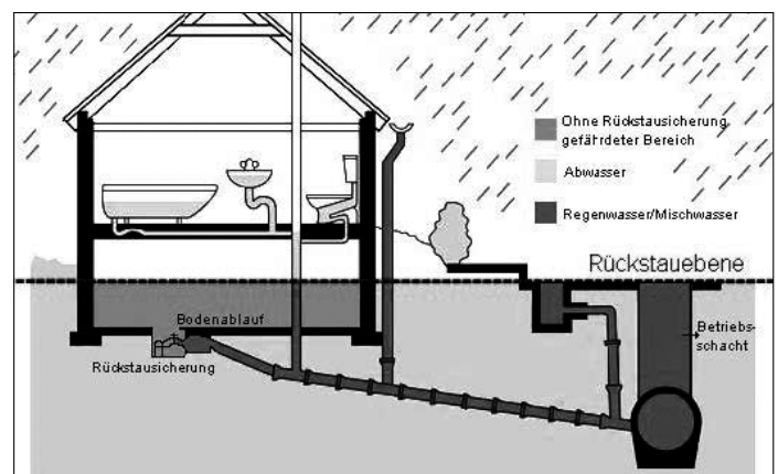
4.2 Rückstauverschlüsse
